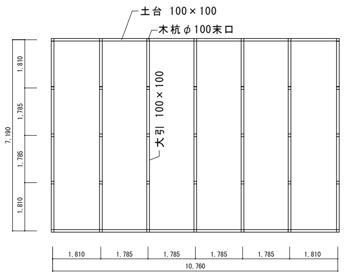
平屋基礎伏図
