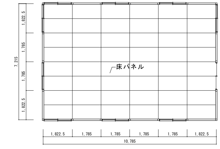
平屋建平面図
